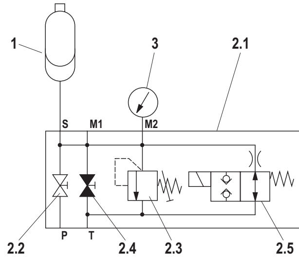
Speicherbaugruppe mit elektromechanisch betätigtem Ablassventil
