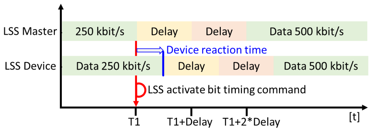
Ablaufdiagramm „Activate bit timing“
