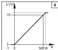
Abb. 2: Spannungsausgang
