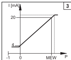
Abb. 1: Stromauegang
