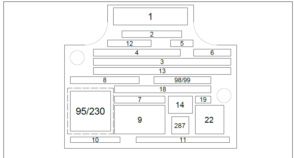
Abb. 3: Typschild DBAW...1X/..6SM..E
