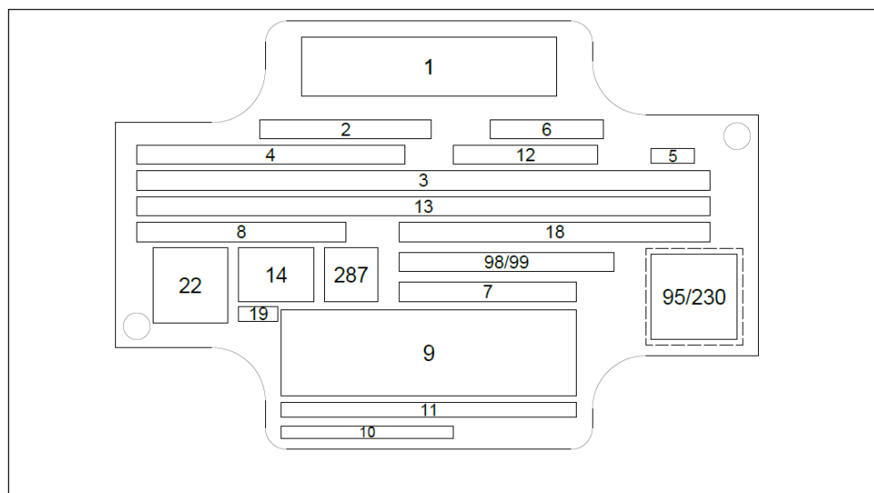
Abb. 2: Typschild DBAW...1X/..6E..E
