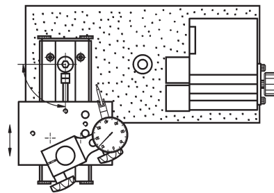
Die Verstellung des Schlittens ist mittels einer Schraube möglich. Die beiden Positionsbohrungen ermöglichen einen vergrößerten Arbeitsraum.
