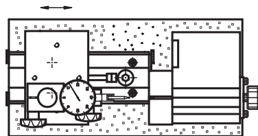
Prüfung eines Innendurchmessers
