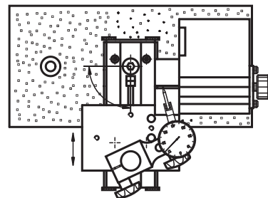
Der Schlitten kann variabel um 90° dreht werden und ermöglicht somit ein schnelles Wegfahren und Positionieren beim Teilewechsel.
