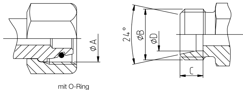
mit O-Ring
