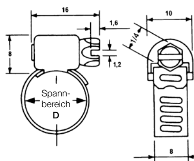
Bandbreite 5/16" - 8 mm
